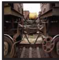
Расцепление
